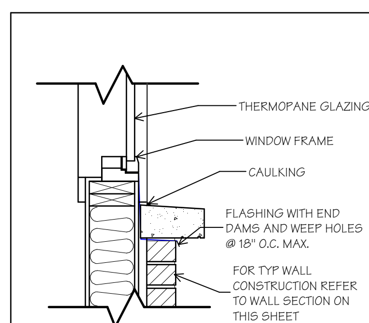
TYP. WIN. SILL SCALE: 1" = 1'-0"
