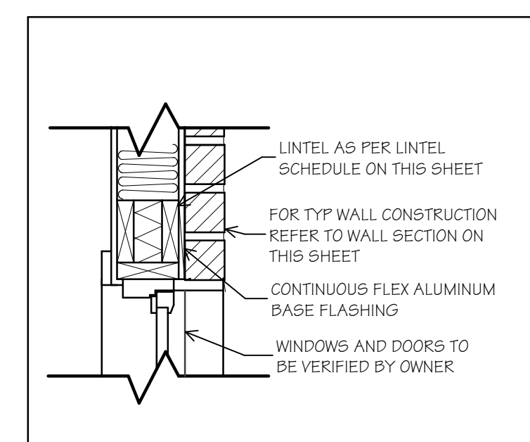
TYP. WIN. SILL SCALE: 1" = 1'-0"
