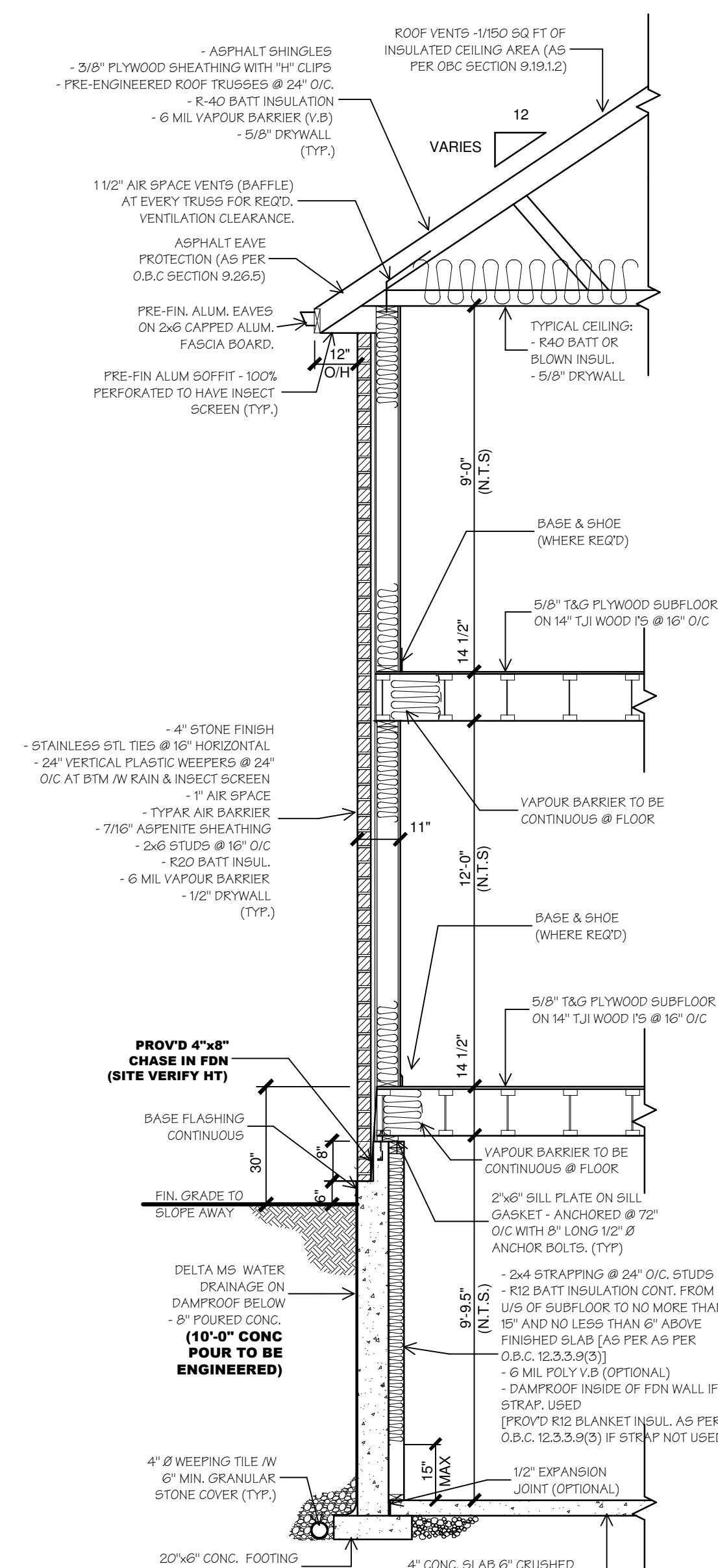
WALL SECTION SCALE: 1/2" = 1'-0"
